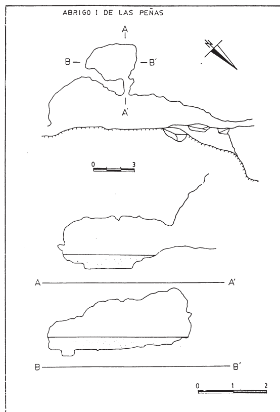
Figura 12. Planta y sección de la cavidad del Abrigo I de las Peñas (PALOMAR, 1982-83).
