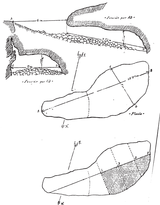
Figura 90. Planta con sectores y secciones de la Cova de la Pastora (BALLESTER TORMO 1949, Fig. 1).
