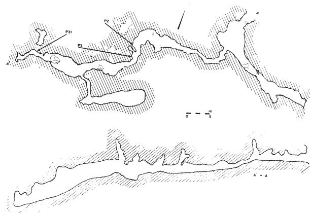
Figura 49. Planta y sección de la Cova Fosca (HERNÁNDEZ y C.E.C., 1988, fig. 213).
