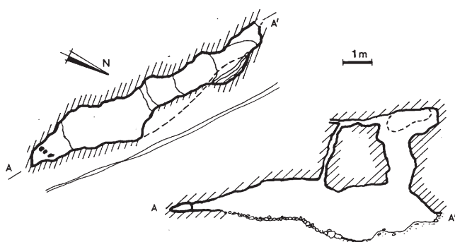
Figura 72. Planta y secciones de la Cova del Negre (PASCUAL BENITO, 1987-88, Fig. 29).
