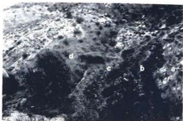
Foto 5.- Contacto entre el Dogger y el Malm donde se observa: a, tramo 3 del Dogger; b, tramo 4 del Dogger; c, tramo 5 del Dogger. Posiblemente y según Azema (1977), sería una transición entre el Dogger y el Malm; d, tramo 1 del Malm. Oxfordiense; e, tramo 2 del Malm.
