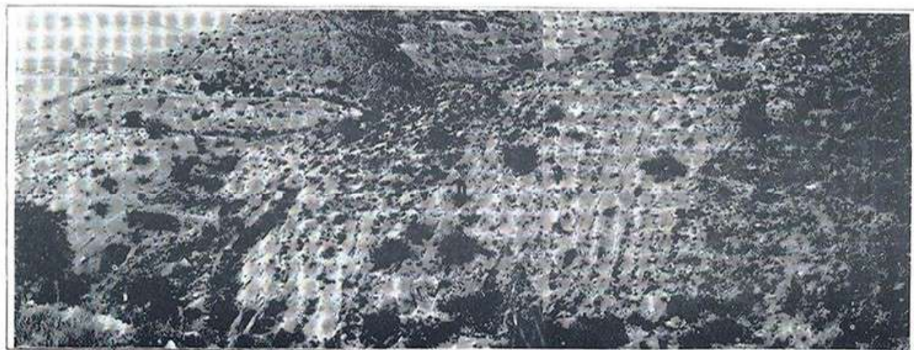
Foto 4.- Vista panorámica del Dogger de La Mola, corte nº 2, así como el contacto con el Lias y el Malm: a, Lias; b, Dogger; c, Malm.
